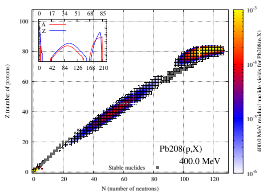
(13.1) 400 MeV
