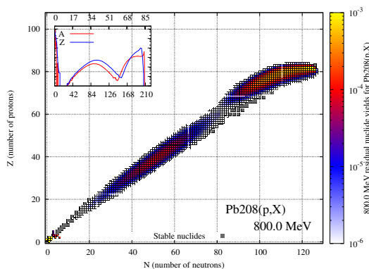
(13.3) 800 MeV
